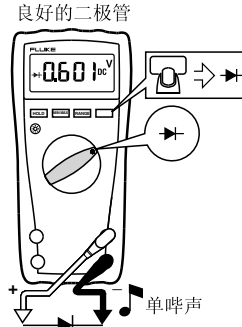
正向偏压
