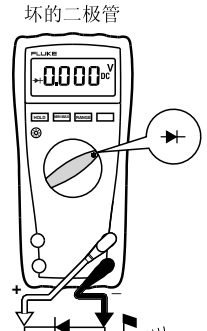
反向偏压
