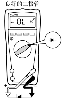
反向偏压
